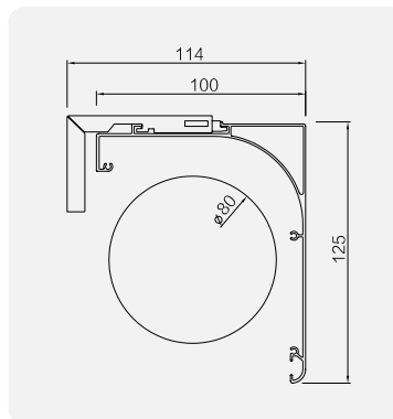
White or Fabric wrapped Z3
